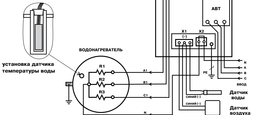
Рис.2 Схема подключения панели управления
